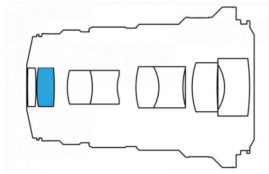
Optischer Aufbau: blau: Low Dispersion Element
