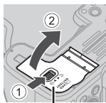
Akku-/Speicherkartenfachabdeckung
