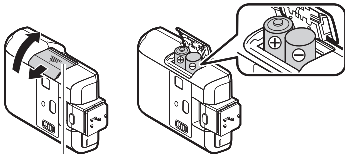
Batteridæksel
