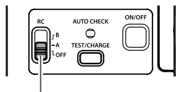
Interruttore RC
