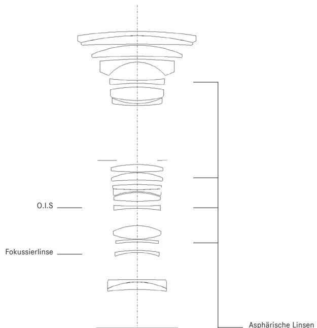
LINSENSCHNITT
