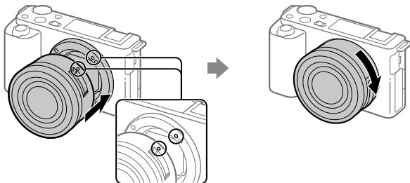
Позначки встановлення
